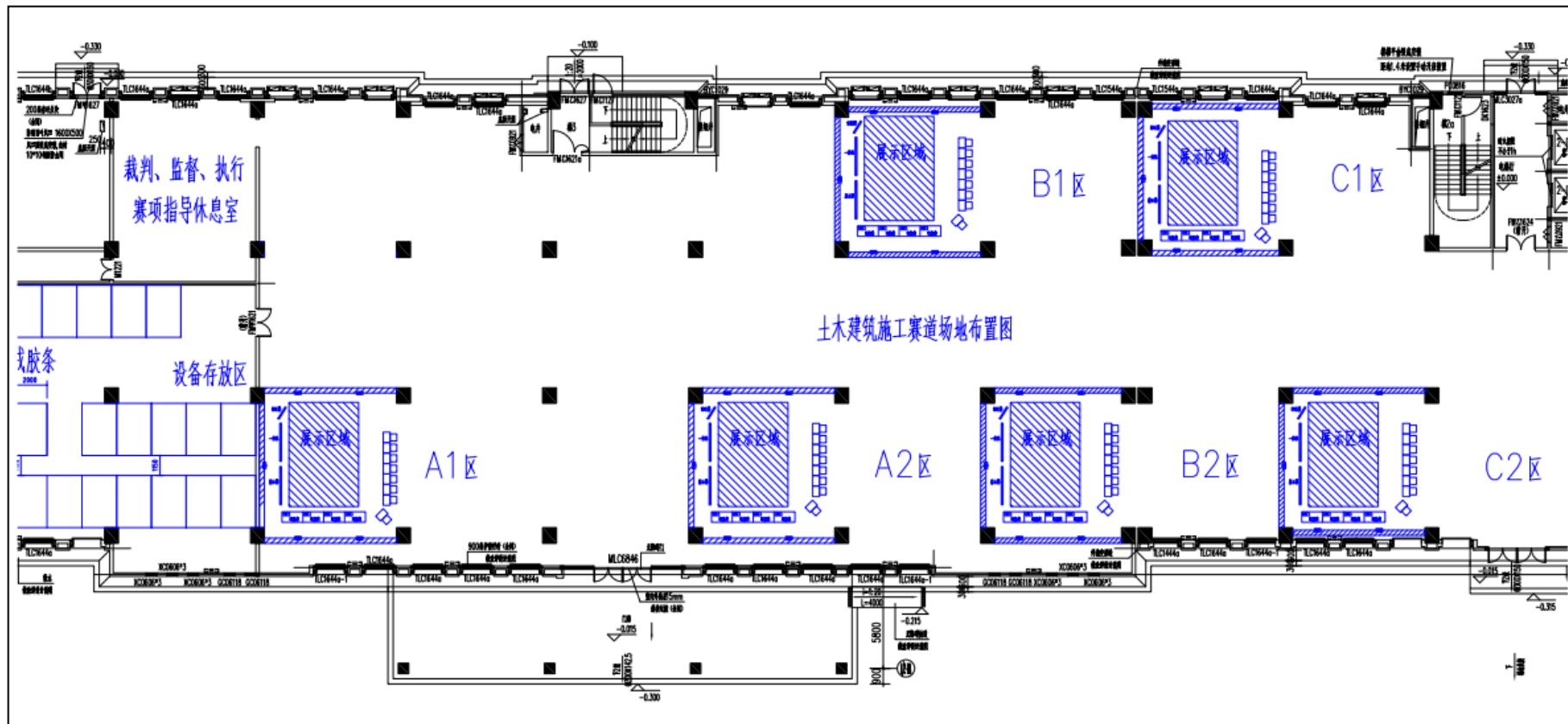
土木建筑施工赛道（高职组）赛布置图
