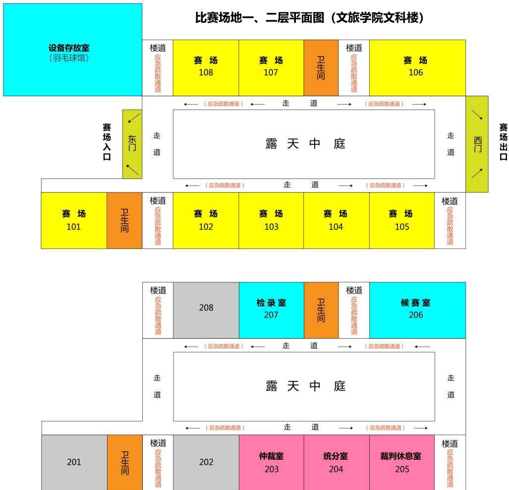
文旅学院文科楼一层、二层平面图
