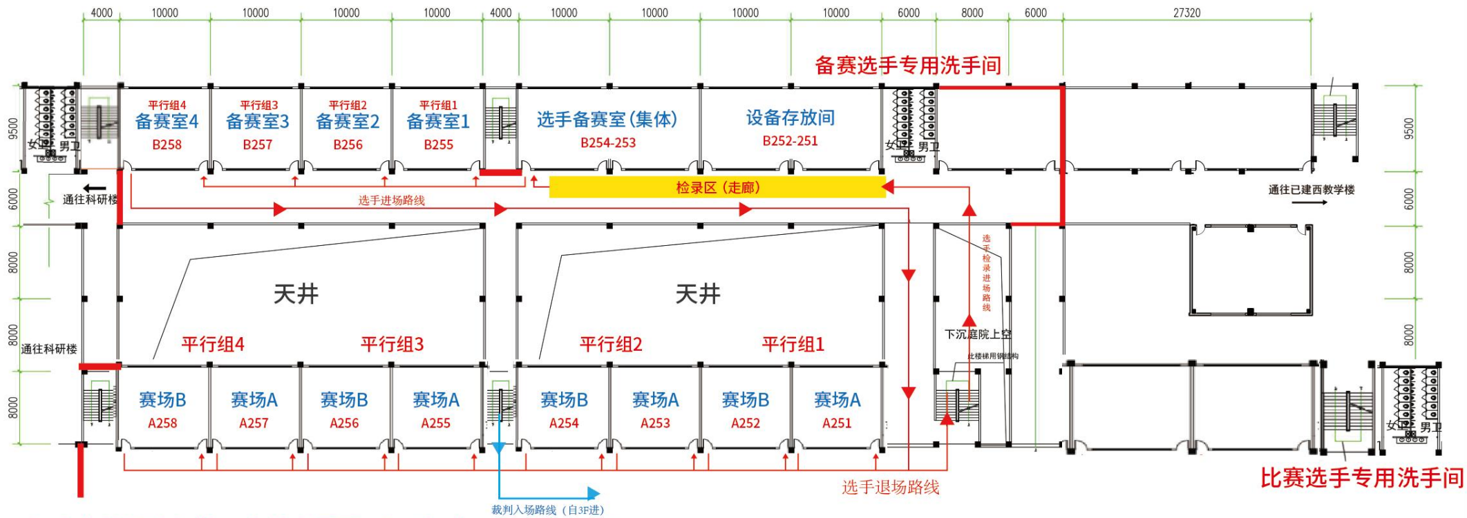
2F 土木建筑设计与管理赛道布局图 (选手仅在2F区域内活动)
